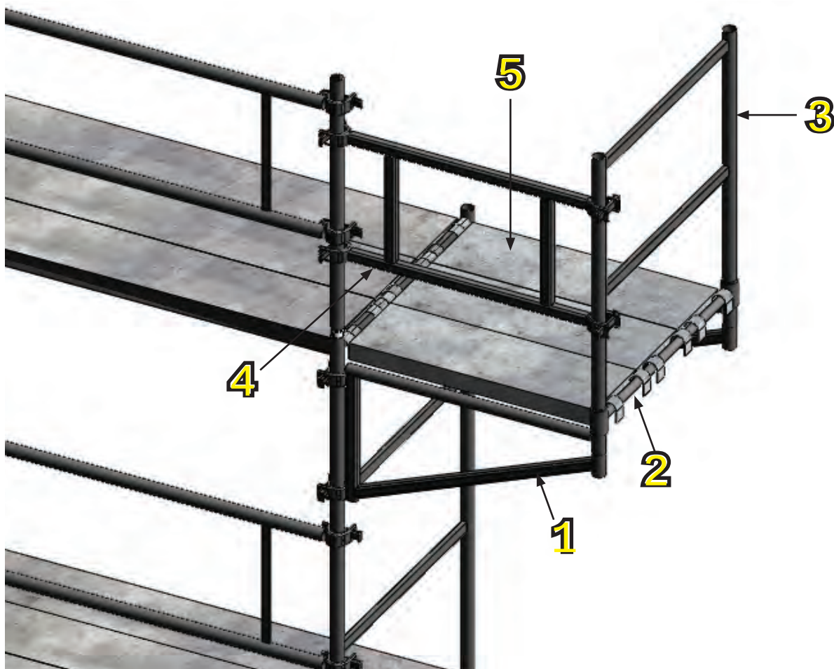
1 Console de déport 1m
